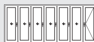
Schéma 761 [1] 6 vantaux pliants-couissants 1 vantail ouvrant à la française
