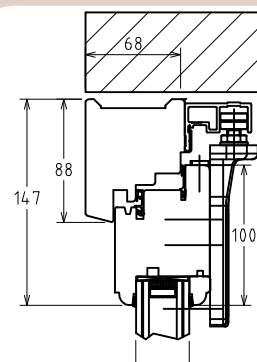
Détail technique appui
