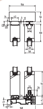
Schéma C 2 vantaux mobiles, 2 vantaux fixes Dessin : montage gauche et droite
