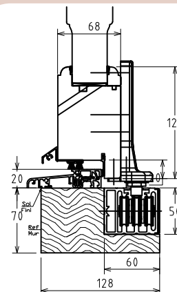
Types de ferrages possibles
