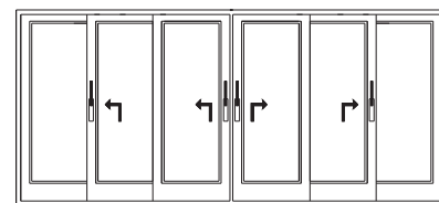
Schéma L 4 vantaux mobiles, 2 vantaux fixes Dessin : montage gauche et droite
