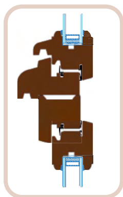
Option : assemblage meneau
