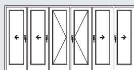
Schéma 633 4 vantaux pliants-couissants 1 vantail semi-fixe, 1 vantail ouvrant à la française
