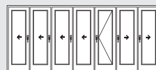
Schéma 743 6 vantaux pliants-couissants 1 vantail ouvrant à la française
