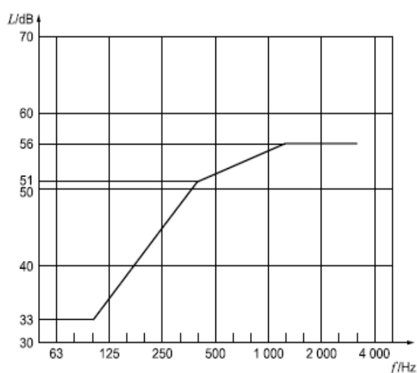
Figure 1 : Courbes de référence pour l'isolement au bruit aérien par bande de 1/3 d'octave
